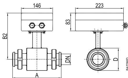
DIN 11851, aufgebaut
