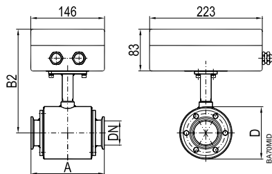
TriClamp®, aufgebaut
